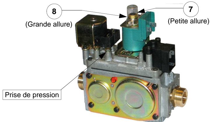
Électrovanne gaz Minigaz Eco 80
